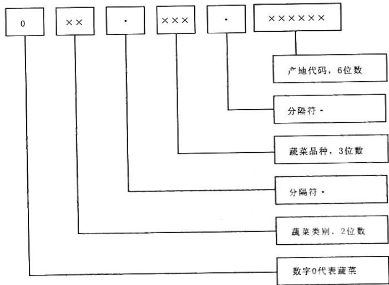
图 1 代码结构
