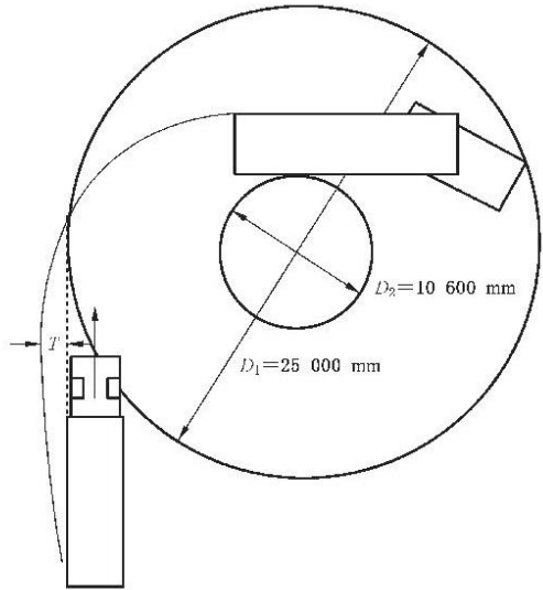
图 B.2 车辆外摆值示意图(汽车列车)
