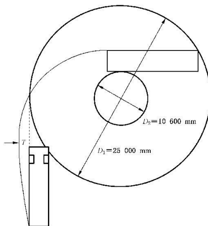
图 B.1 车辆外摆值示意图(汽车)
